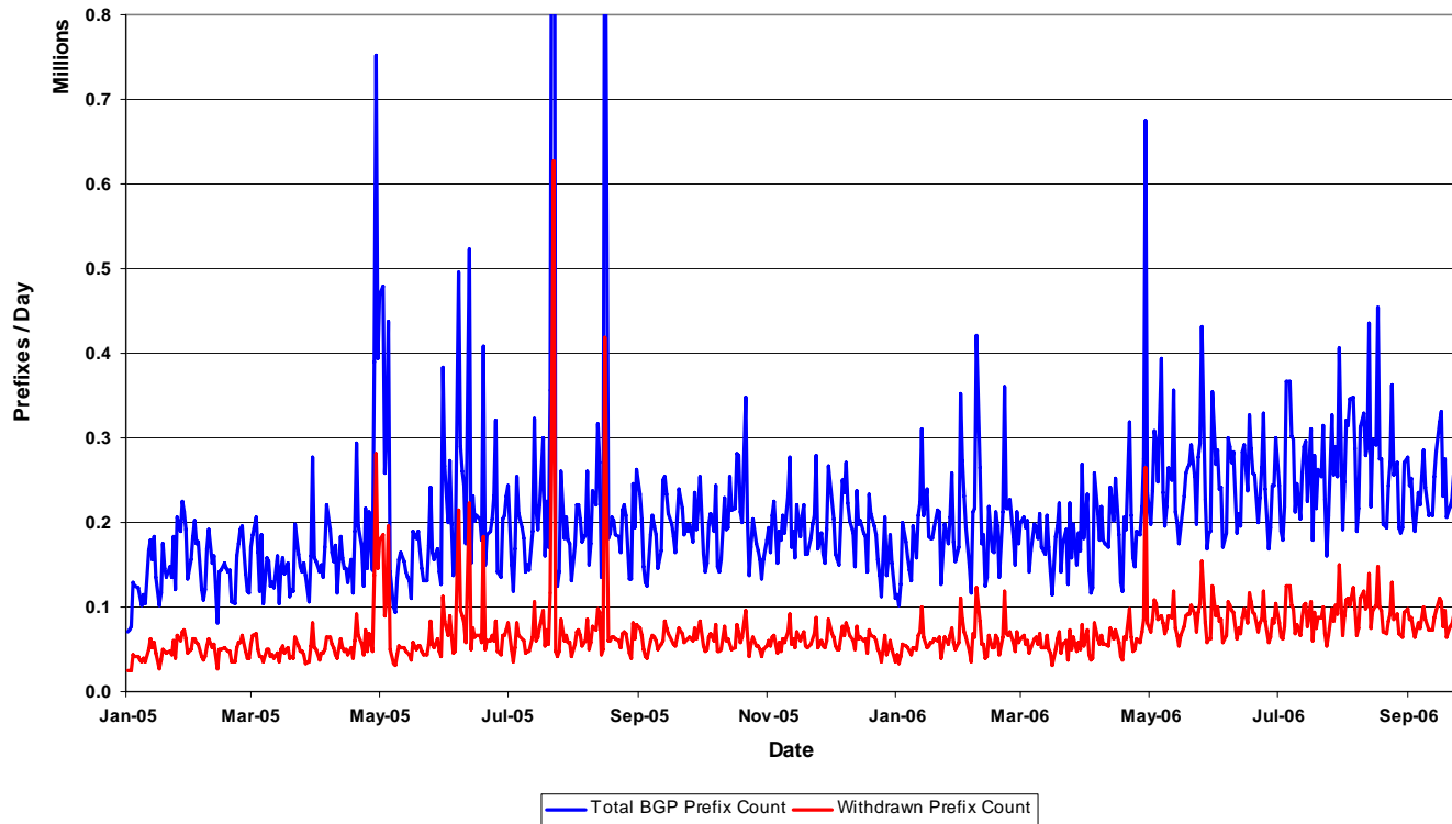
BGP Prefix Updates per Day
